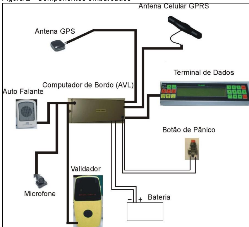
Figura 2 - Componentes embarcados
