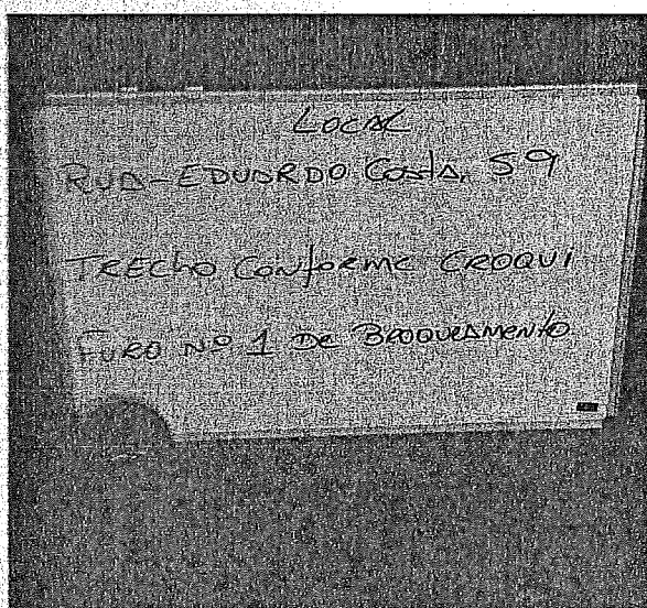
Corpo de prova extraído do Furo nº 1 de Broqueamento com Sonda Rotativa.
