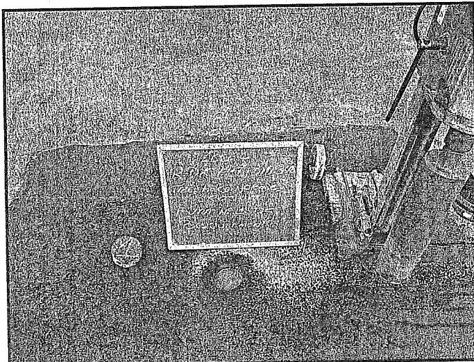
Corpo de prova extraído do Furo N° 1 de Broqueamento com Sonda Rotativa.
